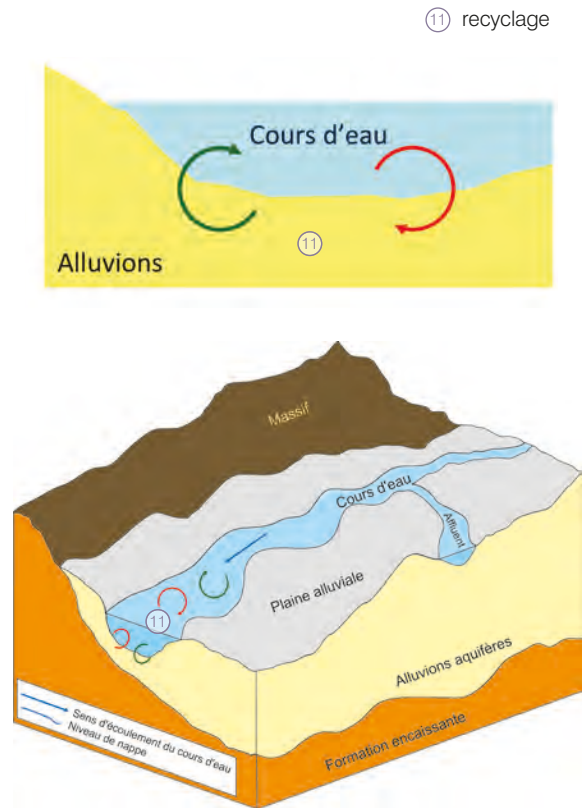
Figure 7. Recyclage d'eau superficielle dans le cours d'eau par exfiltration/infiltration ou échanges hyporhéiques.
