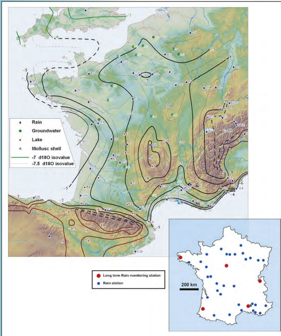
Figure 24. Courbes d'isovaleurs de la composition isotopique de l'oxygène ( \delta^{18}O ) annuelle moyenne des précipitations en France (Millot et al. 2010).
