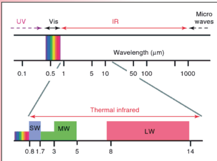
Figure 22. Infrarouge (IR) et régions spectrales adjacentes. L'infrarouge thermique (IRT entre 0,8-14 μm) est composé de l'IR proche (SW shortwave), moyen (MW mid-wave) et lointain (LW long-wave) (Vollmer et Möllmann, 2010).
