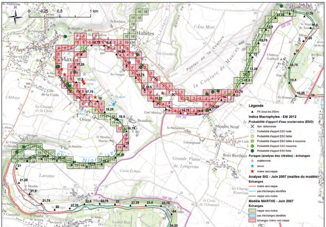
Figure 9. Carte de superposition des résultats de trois diagnostics sur la Sèvre-Niortaise (Fond Scan 25 IGN).
