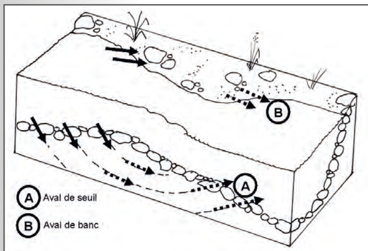
Figure 30. Localisation des zones de remontée potentielle d'eau souterraine vers la surface en aval de seuil et en aval de banc.
