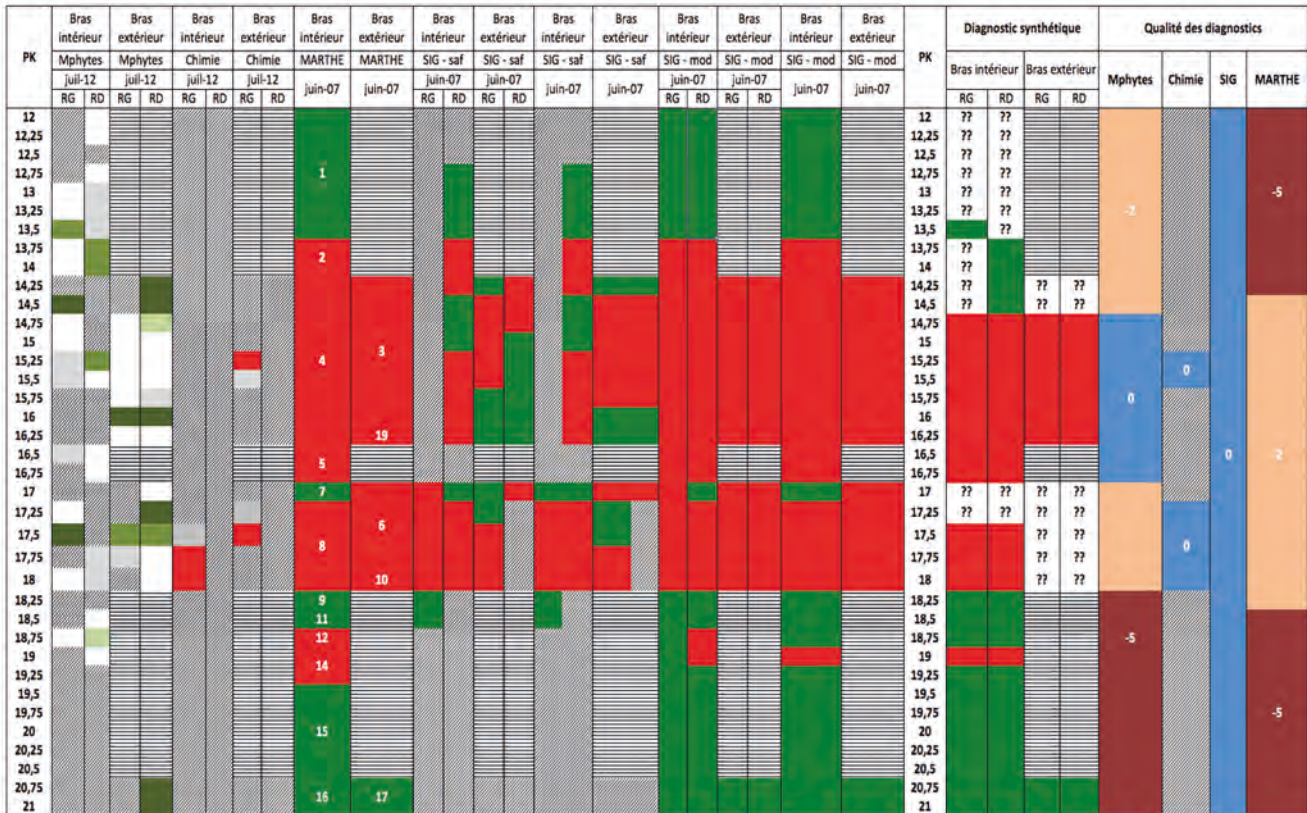
Figure 10. Synthèse croisée des échanges nappe/Sèvre-Niortaise.
