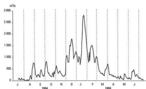
Hydrogramme de la crue à Couzon-au-Mont d'Or
