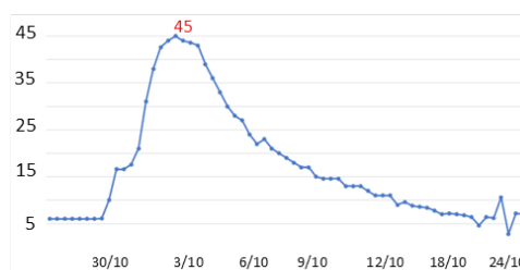
Hydrogramme de la crue de la Tille sur la commune de Cessey-sur-Tille (DDT de Côte-d'Or)
