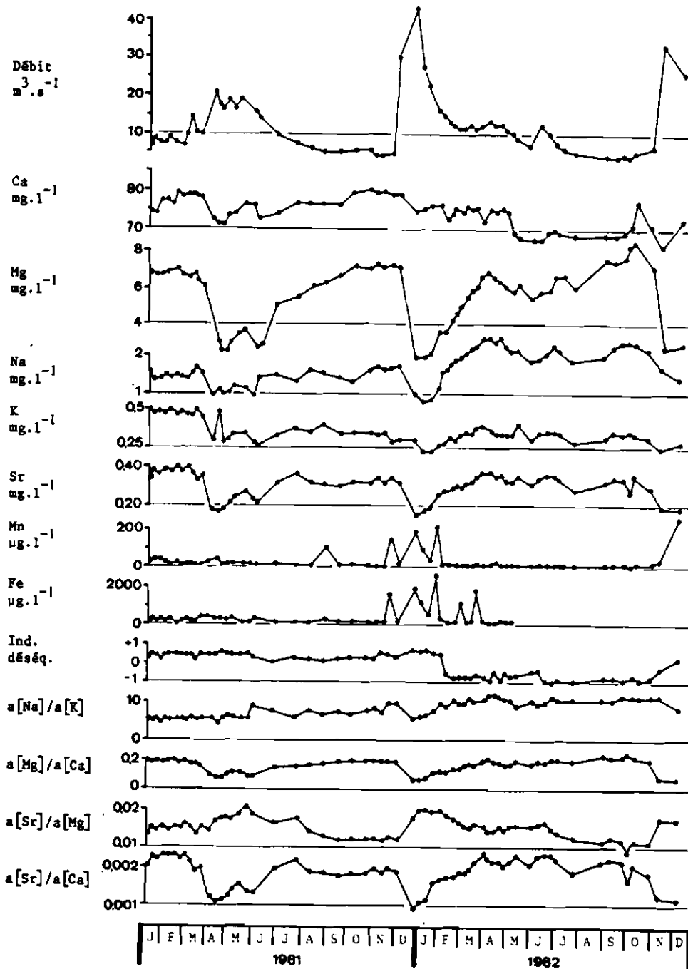
Fig. 52 B : VAUCLUSE HEBOOMADAIRE : VARIATIONS PHYSICO-CHIMIQUES
