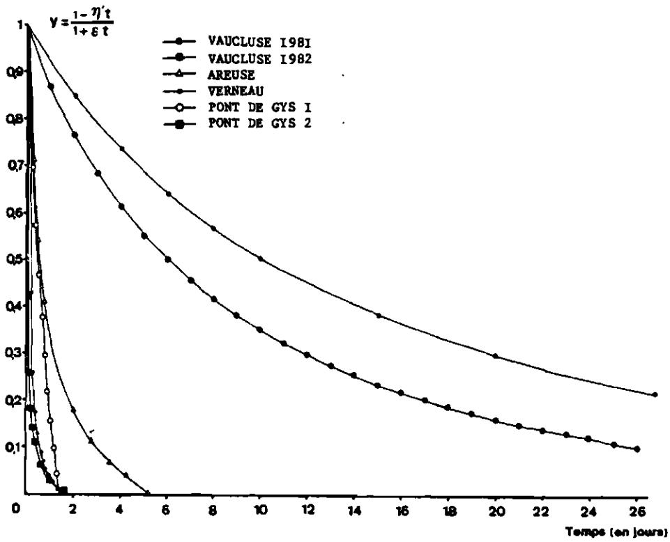
Fig. 145 : COURBES DE DECROU DE L'INFILTRATION : FONCTION Y SUR 4 SYSTEMES KARSTIQUES
