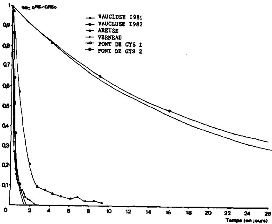
Fig. 146 : COURBES DE DECROU DE L'INFILTRATION, METHODE PHYSICO-CHEMIEUE SUR 4 SYSTEMES KARSTIQUES
