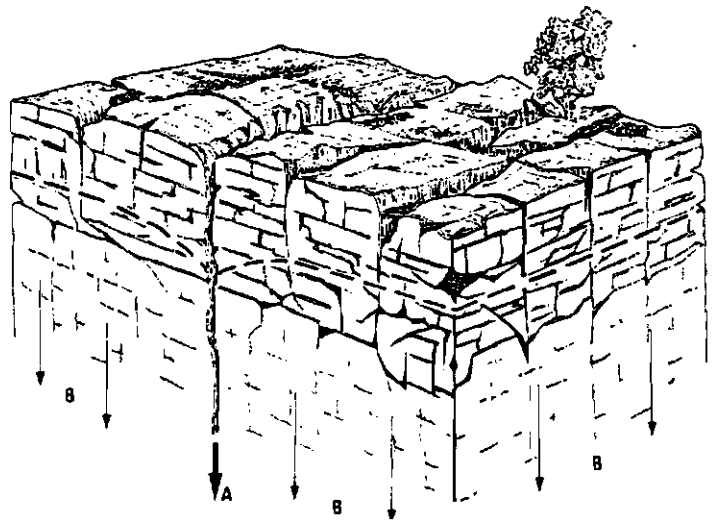
En A est représenté le drainage de cet aquifère vers la profondeur par une fissure largement ouverte. En B est figuré le phénomène d'effluence.
