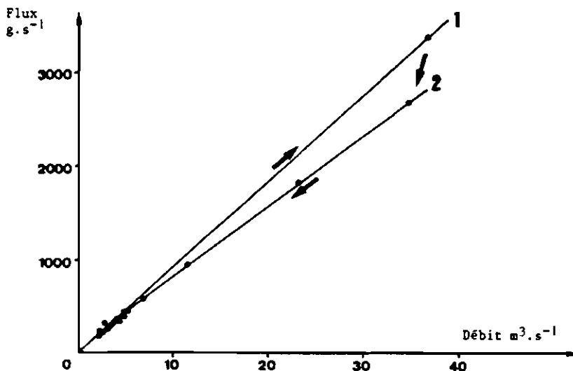
Fig. 123 : RELATION FLUX EN CALCIUM-DÉBIT, SOURCE DE L'AREUSE, CRUE DE NOVEMBRE 1977
