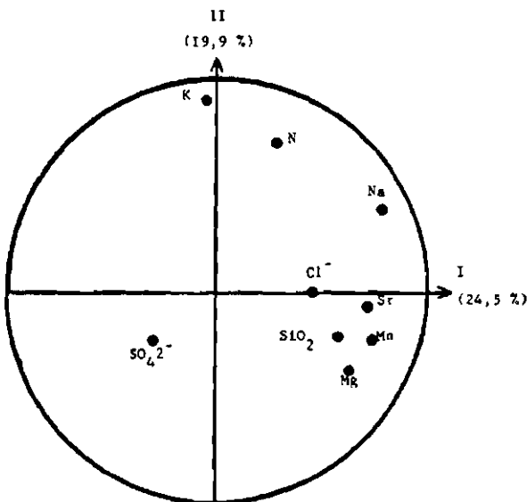
▲ Fig. 97 : BASSES EAUX D'AUTOMNE
