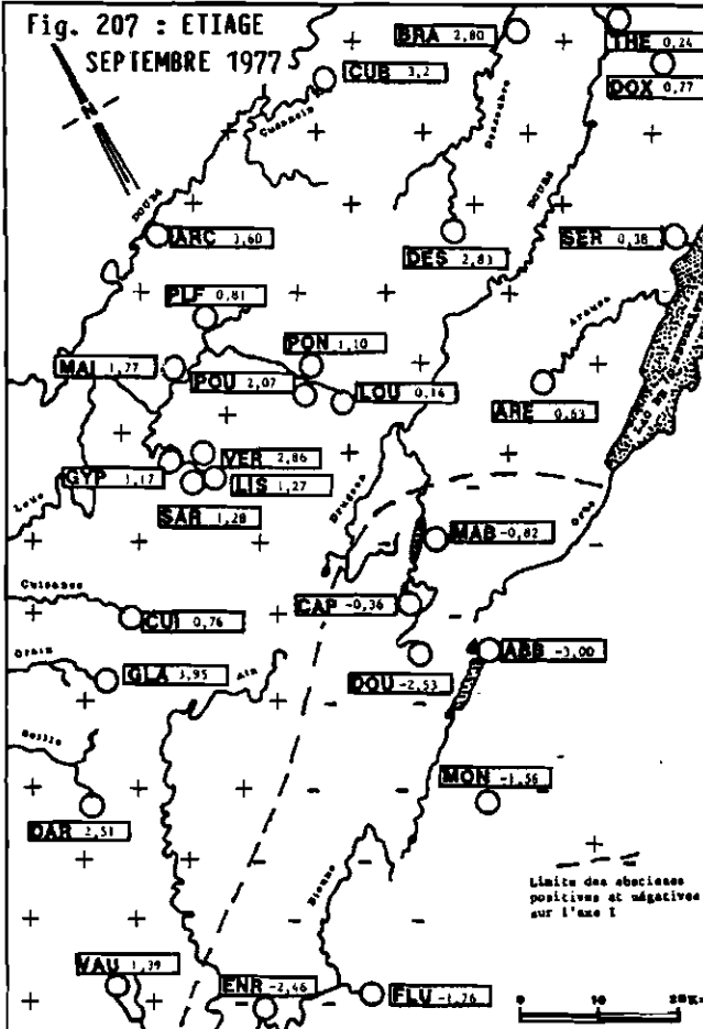
Fig. 205 à 208 : REPARTITION GEOGRAPHIQUE DES ABSCESSES DES EMERGENCES SUR L'AXE FACTORIEL I.
