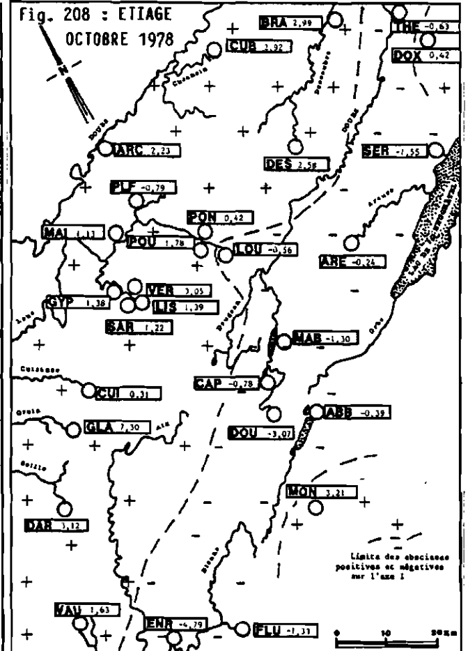
Fig. 205 à 208 : REPARTITION GEOGRAPHIQUE DES ABSCESSES DES EMERGENCES SUR L'AXE FACTORIEL I.
