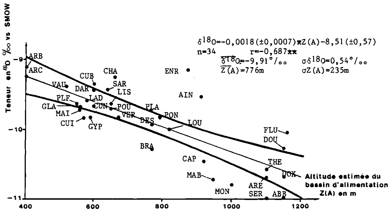
▲ Fig. 171 : QUATRIEME CAMPAGNE : ETIAGE - OCTOBRE 1978
