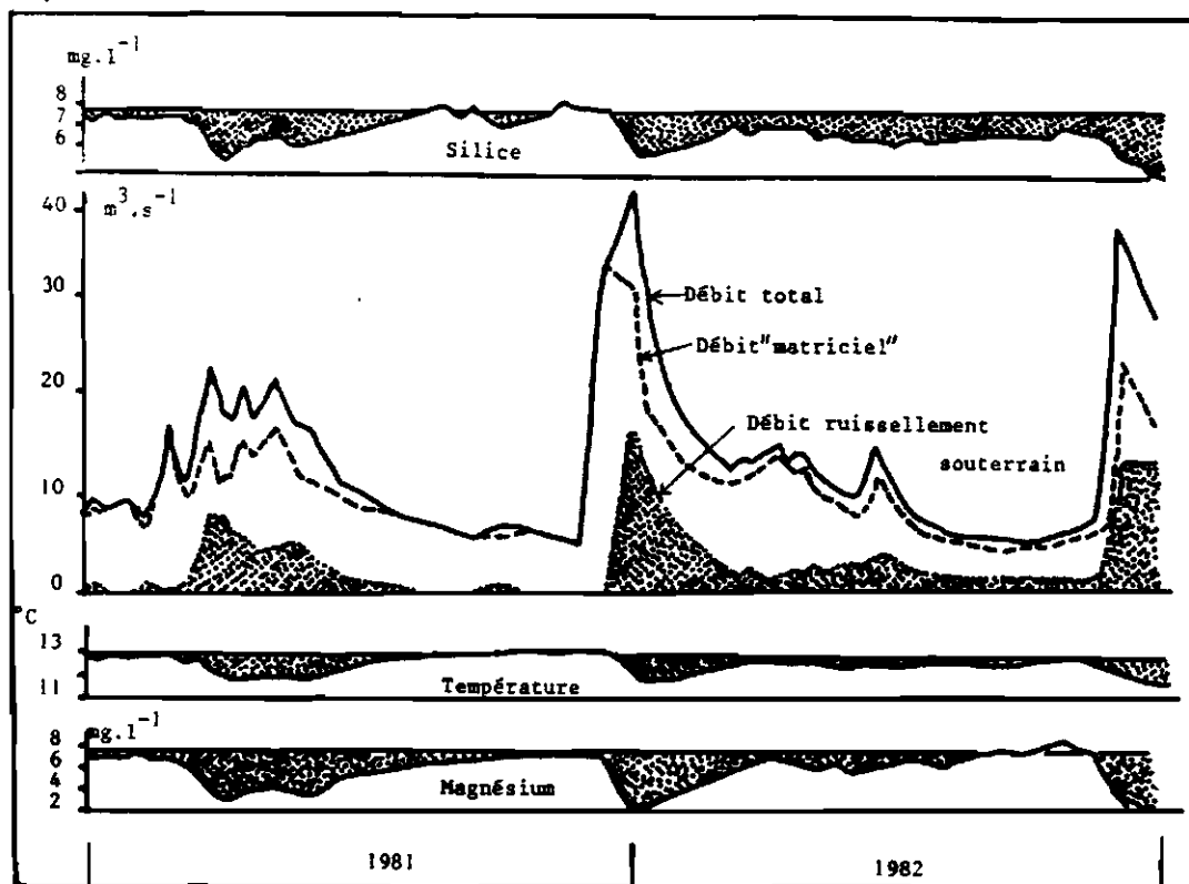
Fig. 140 : DECOMPOSITION D'HYDROGRAMME AVEC LA SILICE - COMPARAISON AVEC L'INFORMATION APPOTEE PAR LE MAGNESIUM ET LA TEMPERATURE
