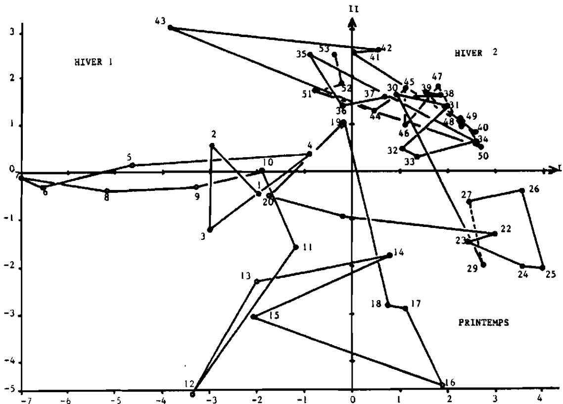
Fig. 67 : LES PLAGNES 1979 - ACP DIAGRAMME DES INDIVIDUS (Plan IxII)
