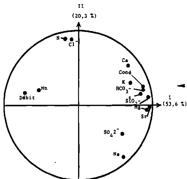
Fig. 78 : VAUCLUSE CRUES HEBOOMADAIRE ACP, DIAGRAMME DES VARIABLES (plan IxII)
